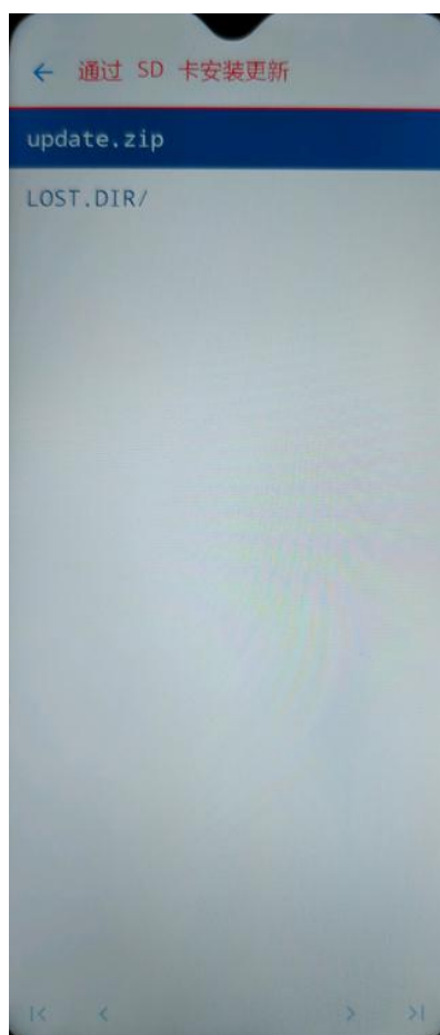
图 3-4 SD 卡目录
